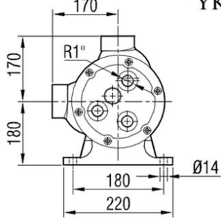
YKF 3"
