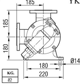
YKF 3"
